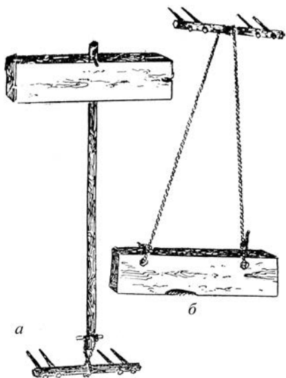
Бороны okly mala (а) и yüpli mala (б) (по: Очерки по истории хозяйства и культуры туркмен, 1973. С. 19)
