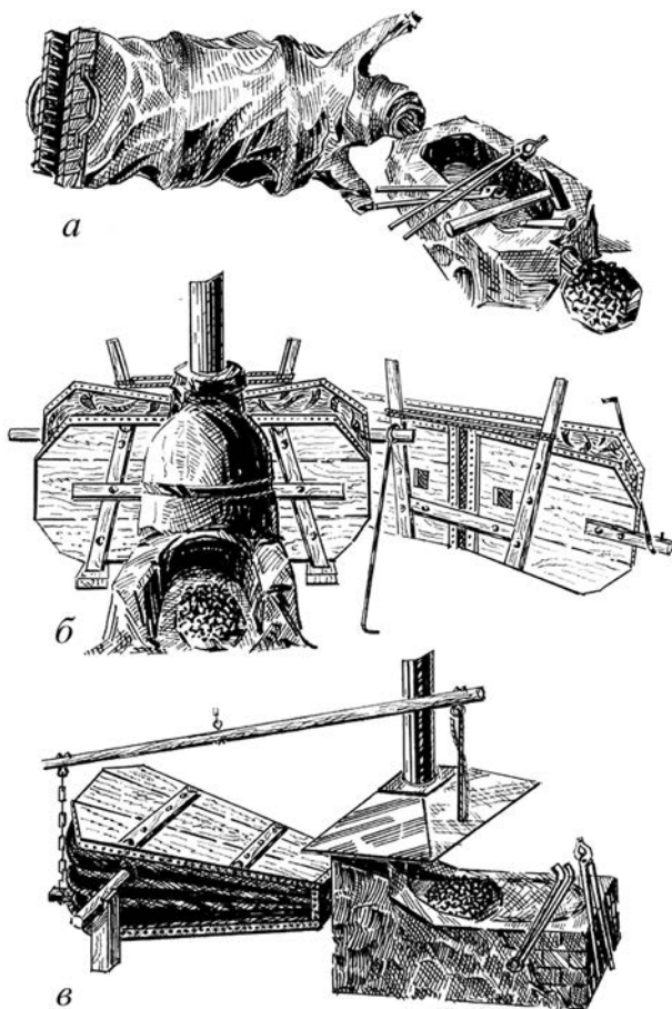
Кузнечные горны и меха: а) раннего периода; б) более позднего; в) современные Рисунок А. Долгова
