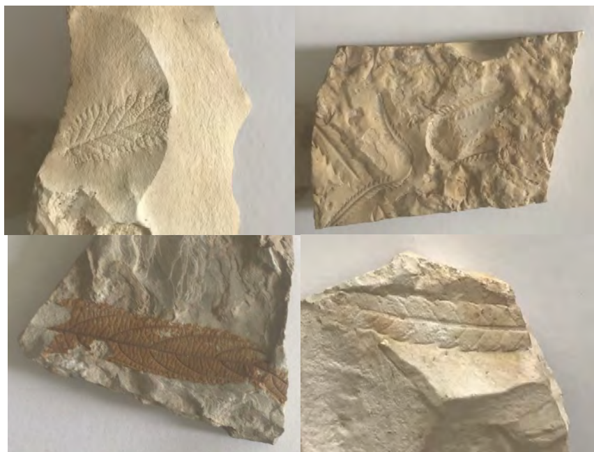
Отпечатки эоценовых растений из Еройландуза. Из личной коллекции Ю.К. Горелова.
